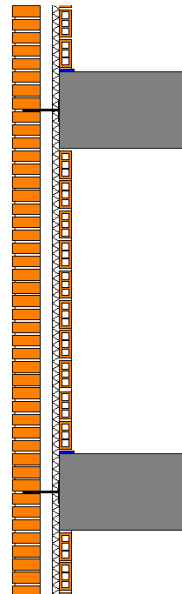
Fachada Structura autoportante y ventilada
