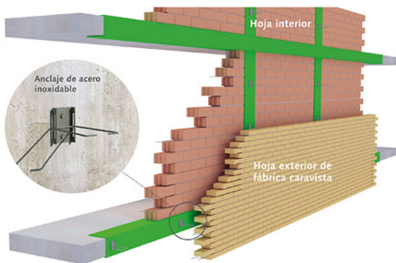
Fachada Structura autoportante y ventilada
